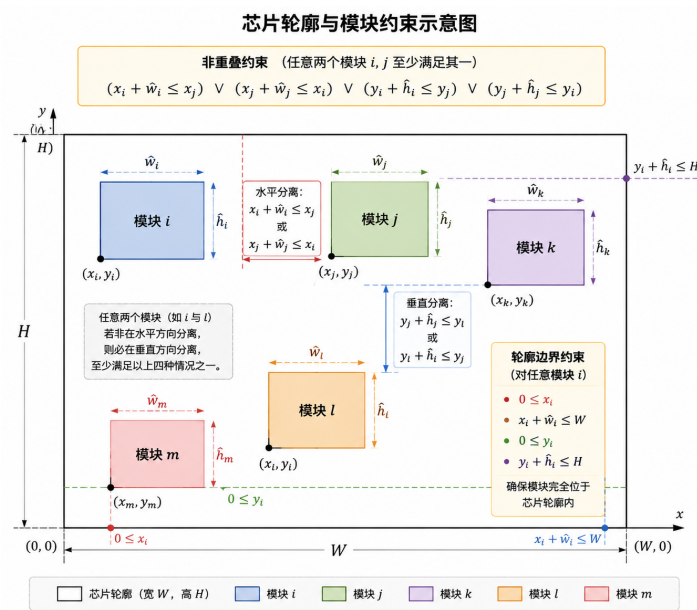
图 2 问题一约束条件示意图
